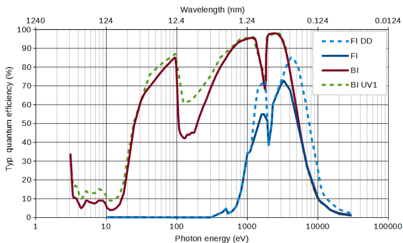
Кривые квантовой эффективности QE серии ALEX-s
