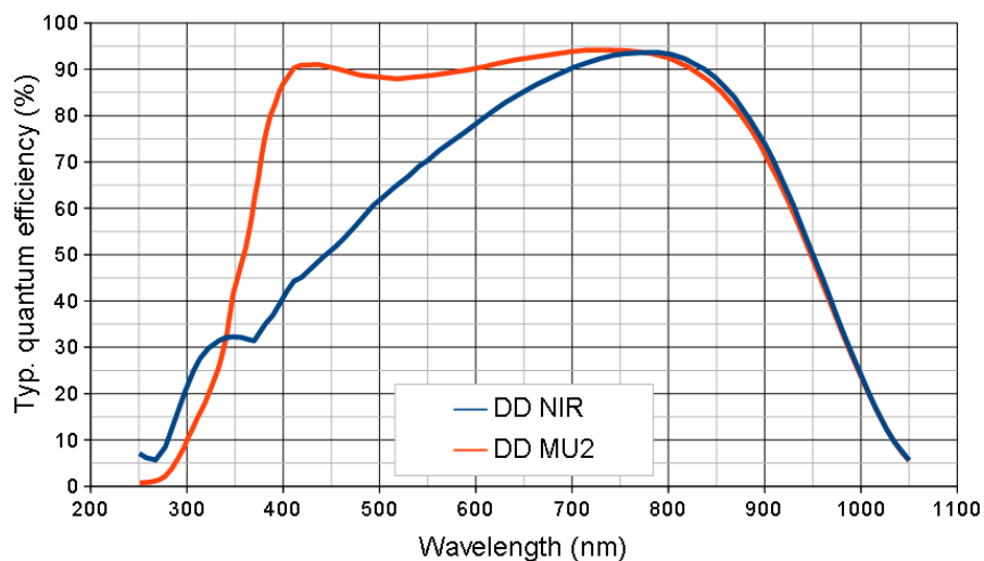
Кривые квантовой эффективности ПЗС-датчики NIMO с глубоким истощением для диапазона NIR
